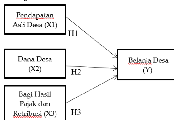
Gambar 1. Kerangka Penelitian
